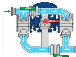
2Q — ПАРАЛЕЛЬНО
